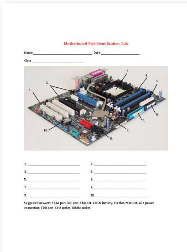
Figura 29. Identificación de las partes de una tarjeta madre de un computador (crédito: https://www.scribd.com/doc/ ).
